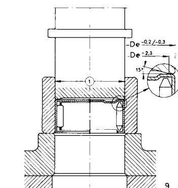
(1) Diametro interno bussola di guida: (De + 0,3) mm.
